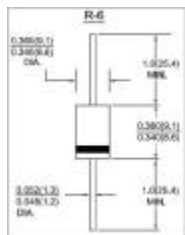
R-6
