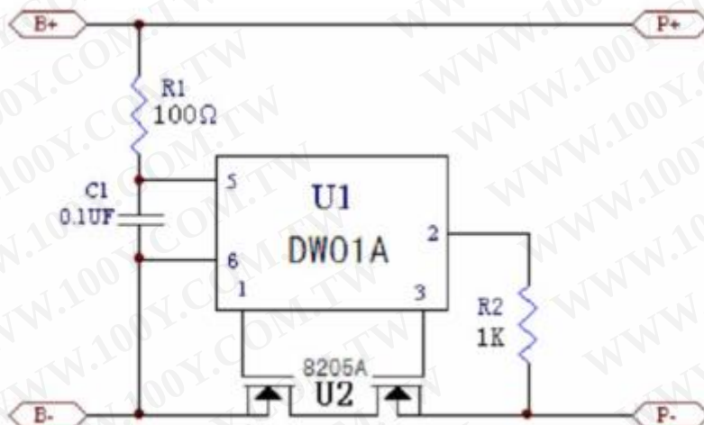
7.4 Circuit Diagram 原理图
