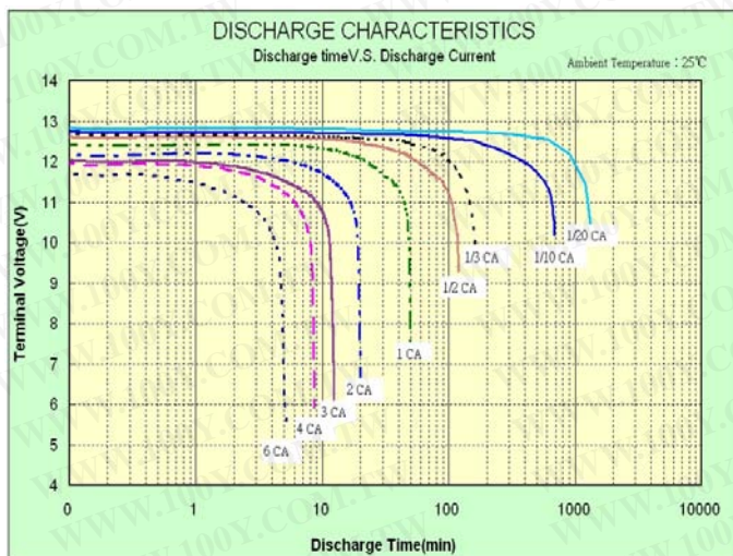
1. 放電時間與放電電流的關係 (Discharge Time VS Discharge Current)
