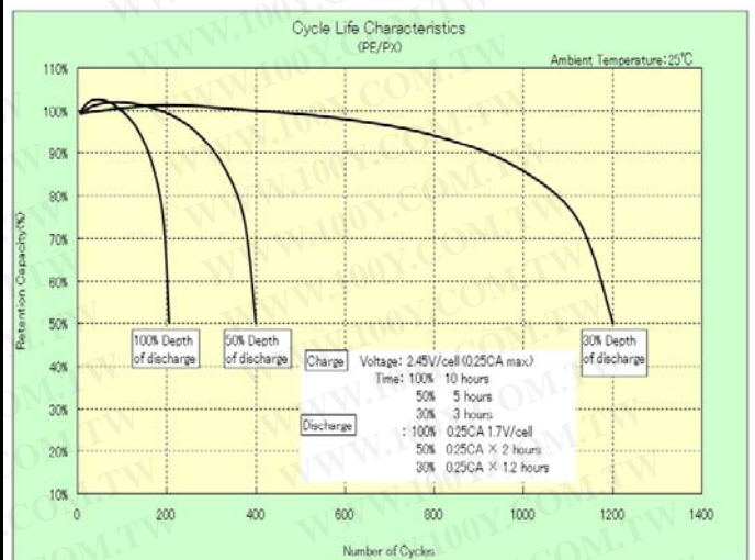
2. 循環使用壽命之特性 (Life Characteristics of Cycle Use)
