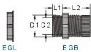
EGL 螺帽 EGB 本體和夾緊爪
