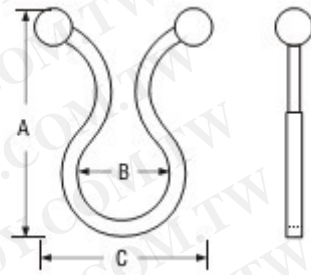
電線束線環 TT 系列工程圖
