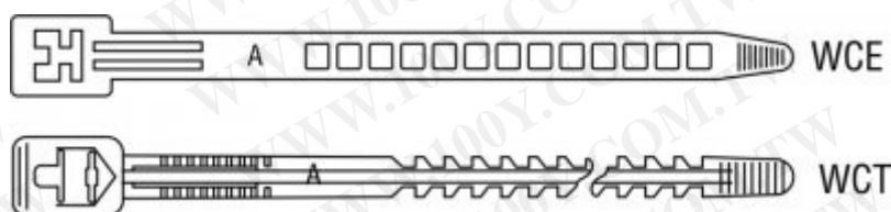
電源線束線帶 WCE 系列產品工程圖
