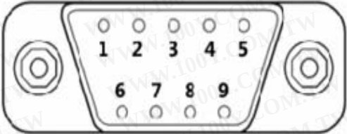
DB9公头（针）
