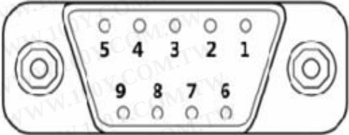
DB9母头（孔）
