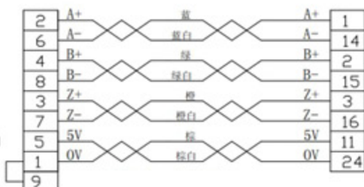
配线图
