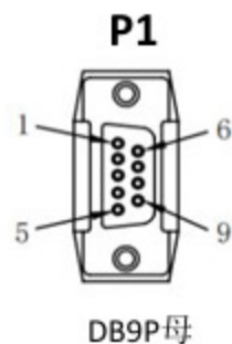
P1 DB9P母
