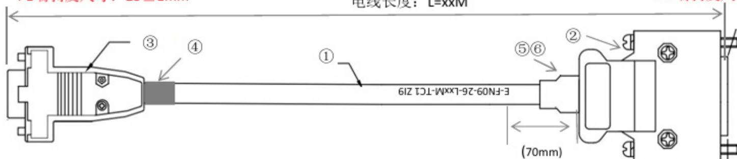
配线图
