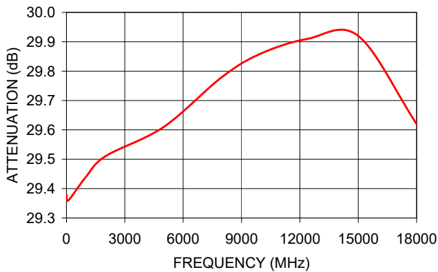
BW-S30W2+ ATTENUATION
