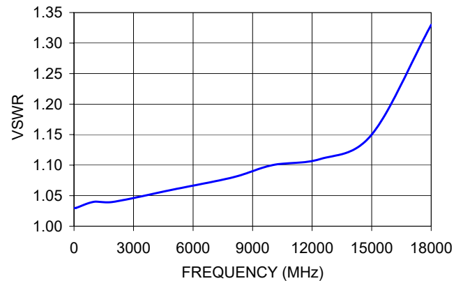
BW-S30W2+ VSWR
