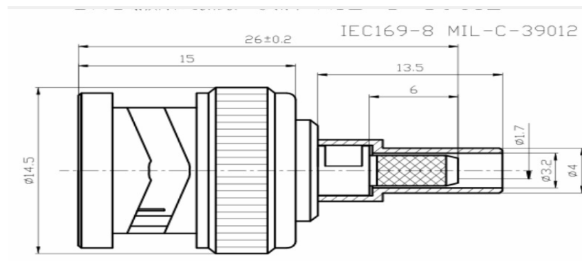
BNC-J 接頭
