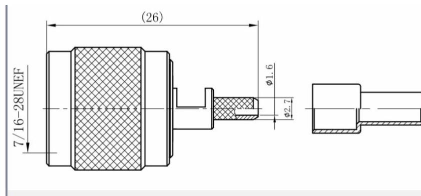
TNC-J 接頭
