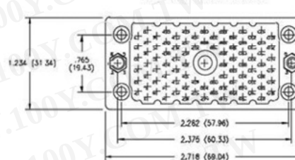
90 PIN RECEPTACLE
