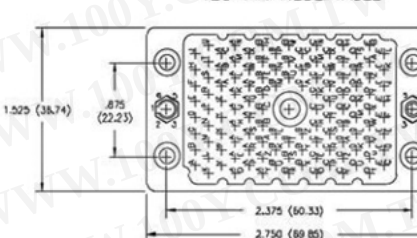
120 PIN RECEPTACLE
