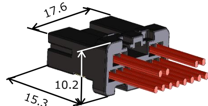
<Plug> ZE05-12DS-HU/R
