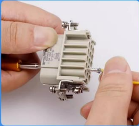
3、平缓地将端子推出
