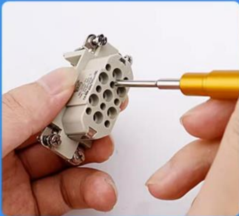
1、选择合适的退针工具，并对准要取出的端子
