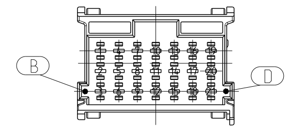
CODING C (GROOVES B-D) (Nuten B-D) SHOWN AS EXAMPLE als Beispiel gezeigt
