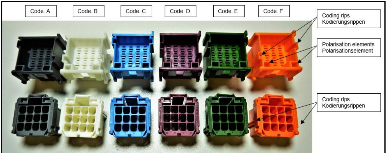
Figure / Abbildung 3.5.1.1 Exemplarily: 12Pos. controlling of coding and polarisation. Beispielhaft: 12Pol. Abfrage Kodierung und Polarisierung.
