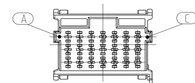
CODING B (GROOVES A-C) (Nuten A-C) SHOWN AS EXAMPLE als Beispiel gezeigt
