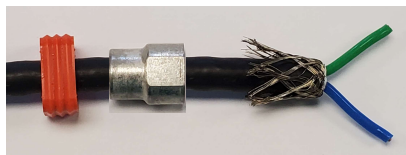
Figure / Abbildung 3.1.5.1: Separation of single wires / Vereinzelung der Einzelleiter
