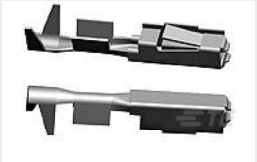
TE Part #1355717-5 MQS0,63 Au rec LL unseal. 0,08-0,22
