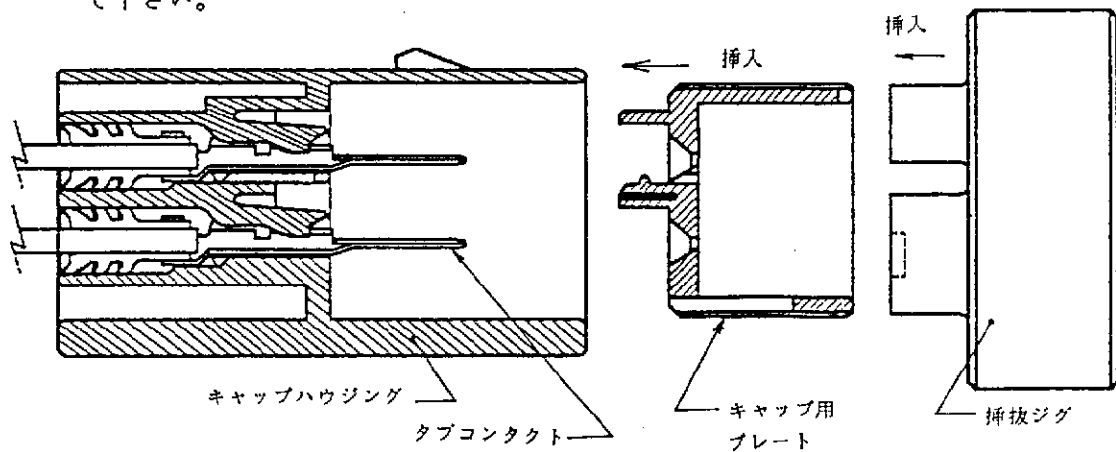
図3. キャップ用プレートの装着
