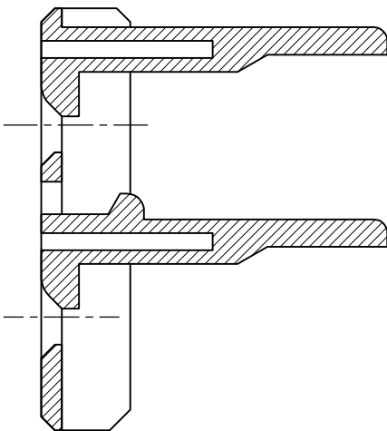
SECTION 断面 A-A (尺度 5:1)
