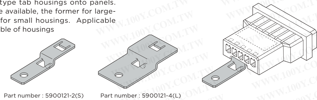
Part number : 5900121-2(S) Part number : 5900121-4(L)
