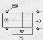
Montageausschnitt/Panel cut-out
