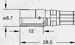
Buchsenkontakt/Socket contact
