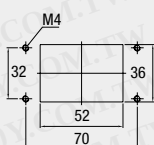
Montageausschnitt/Panel cut-out
