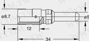
Stiftkontakt/Pin contact
