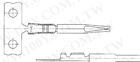
Socket
