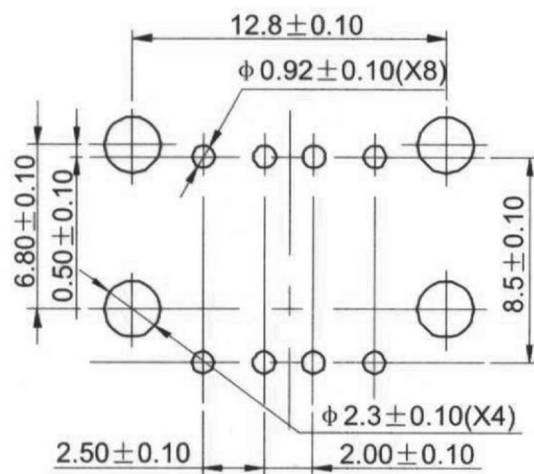
P.C.B LAYOUT
