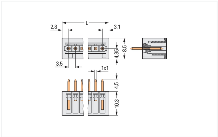
外形尺寸 (单位 : mm) L = (极数 - 1) x 焊针间距 + 5.9mm
