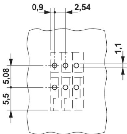
开孔图/焊盘环宽
