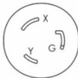
L6-20P
