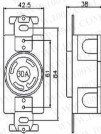
尺寸圖 Dimension
