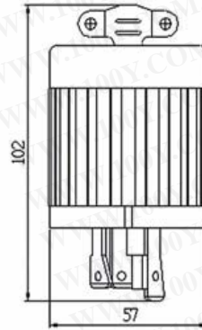
尺寸圖 Dimension
