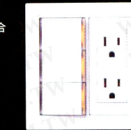
WTDFP4932K 埋入式開關+插座2連組合 (附螢光開關C(參)+ 接地極雙插座)(附蓋板) 開關 15A 110V AC用 插座 15A 125V AC
