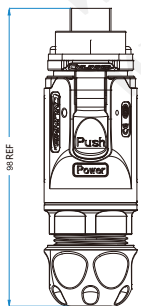
产品外型尺寸图 dimensions figure
