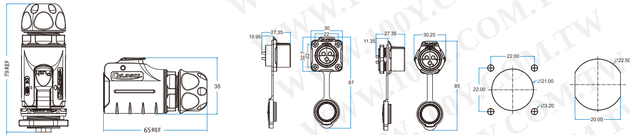
产品外型尺寸图 dimensions figure
