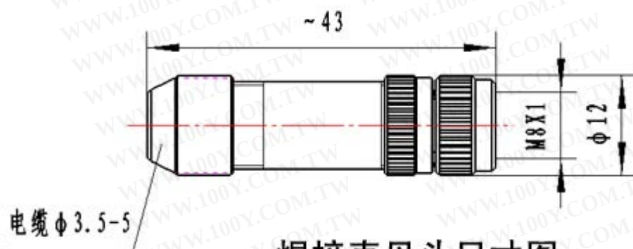
焊接直母头尺寸图
