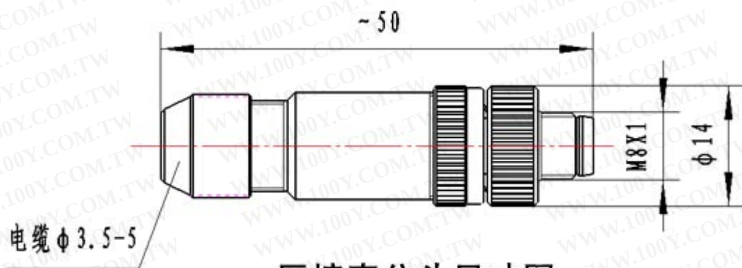
压接直公头尺寸图
