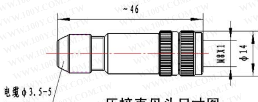
压接直母头尺寸图
