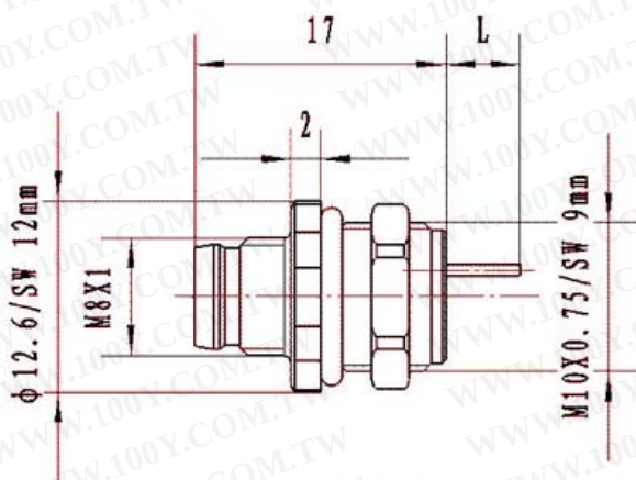
尺寸图
