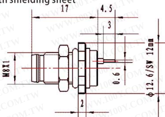
尺寸图
