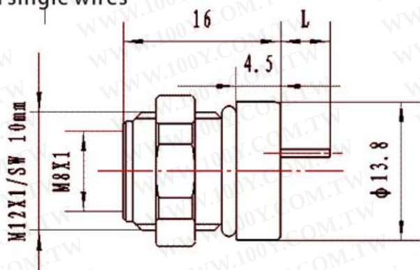
尺寸图
