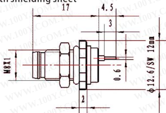
尺寸图
