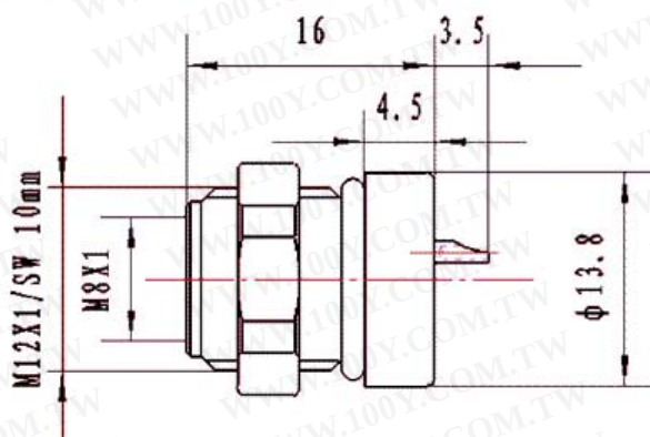
尺寸图
