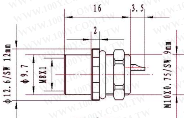
尺寸图
