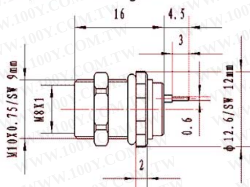
尺寸图
