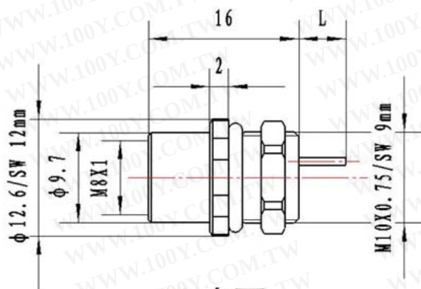
尺寸图
