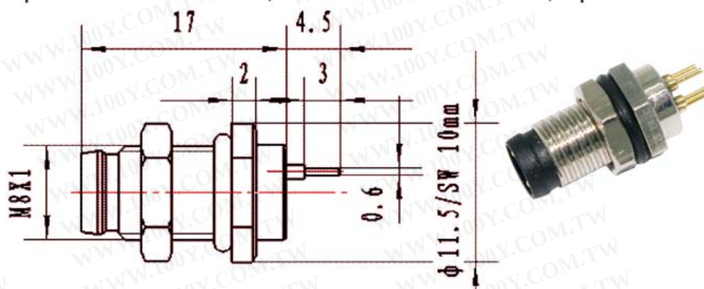
尺寸图
