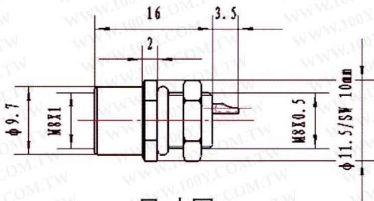
尺寸图
