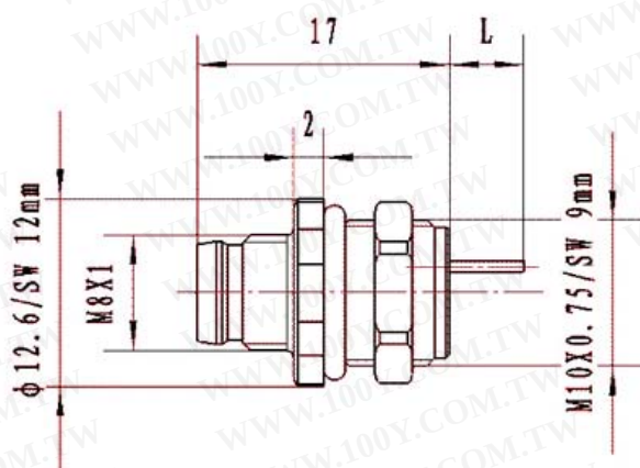
尺寸图
