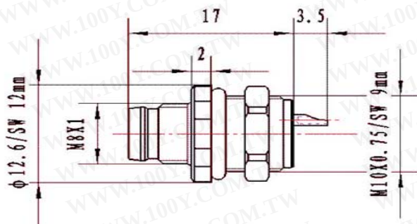
尺寸图
