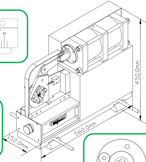
压接机构
