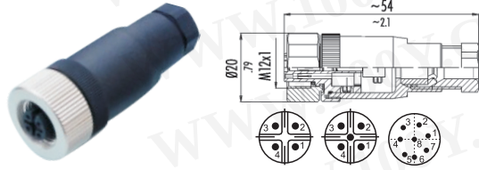
M12直母头（可选A/B/D型）
