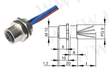
M12插座(孔, M16*1.5 焊线式后板安装
