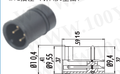
尺寸图 Drawing
