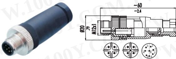
M12直公头（可选A/B/D型）
