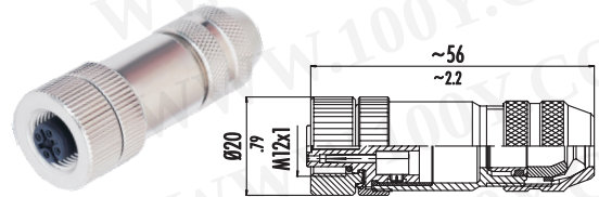
M12屏蔽直母头（可选A/B/D型）
