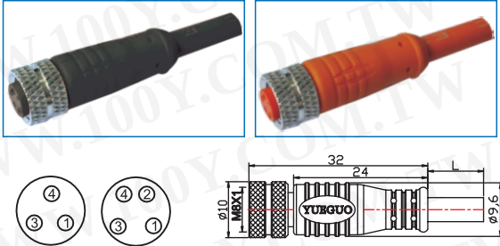
M8电缆直母头
