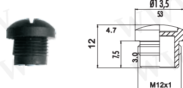
M12母座防护盖
