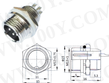
MI2插座 (针, MI2+1 PCB后极安表)
