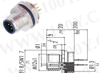
M12插座 (针, M16*1.5 PCB后板女表)
