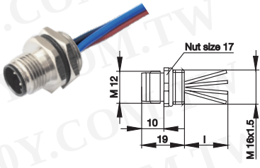
M12插座(针, M16*1.5 焊线式后板安装)
