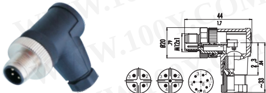
M12弯公头（可选A/B/D型）
