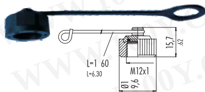
M12公座防护盖（带绳）
