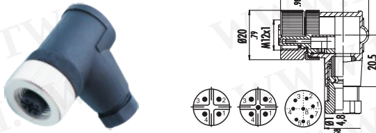
M12弯母头（可选A/B/D型）
