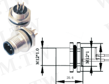
MI2插座 (针, MI2+1 PCB后极安表)
