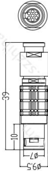
护套型插头
