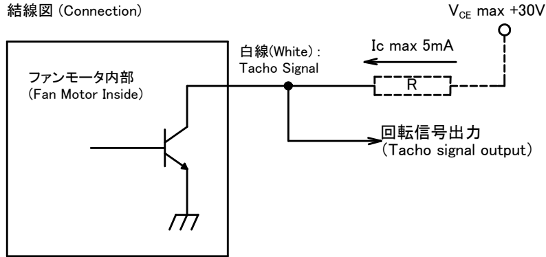
結線図 (Connection)
