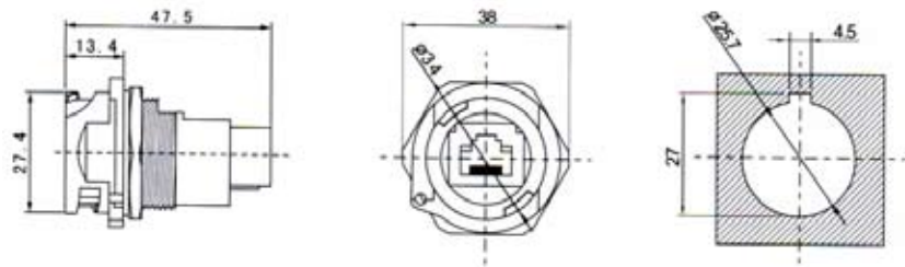
RJ45 Socket 防水面板安裝插座 (含防塵蓋) 型號：RJ45F71
