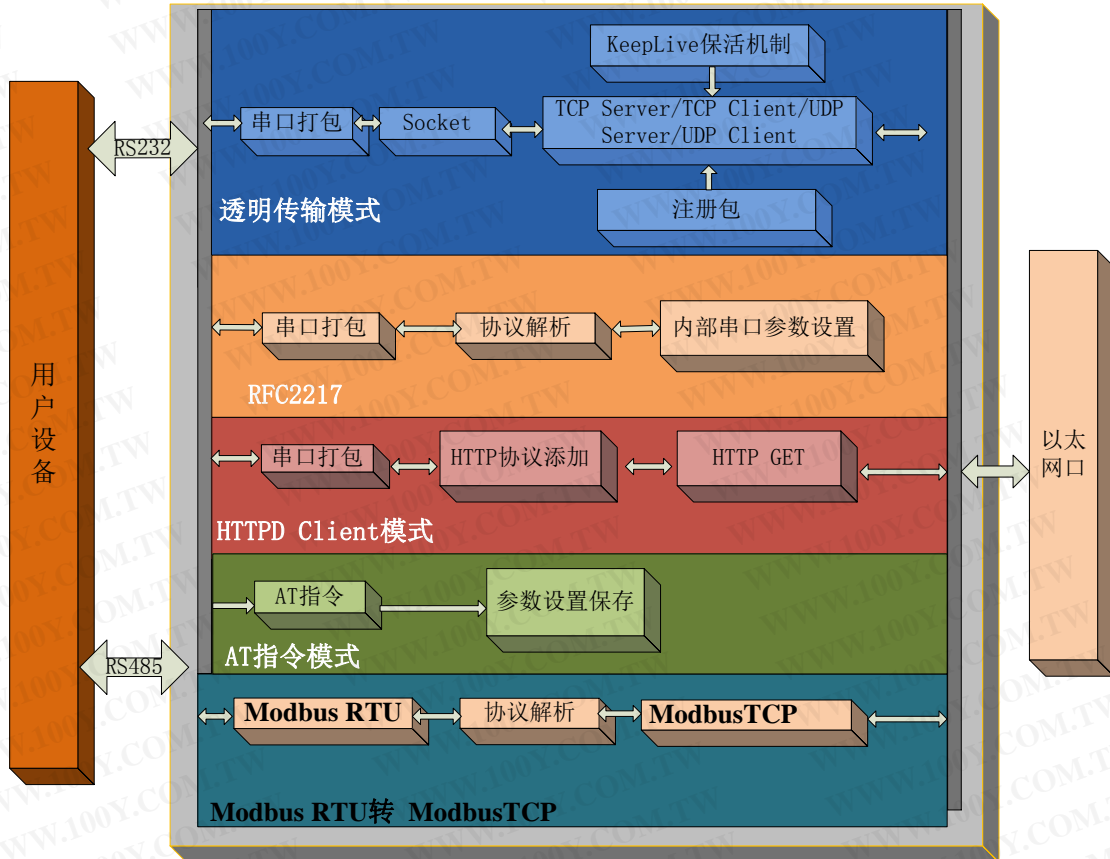
图 5 410S 功能框图
