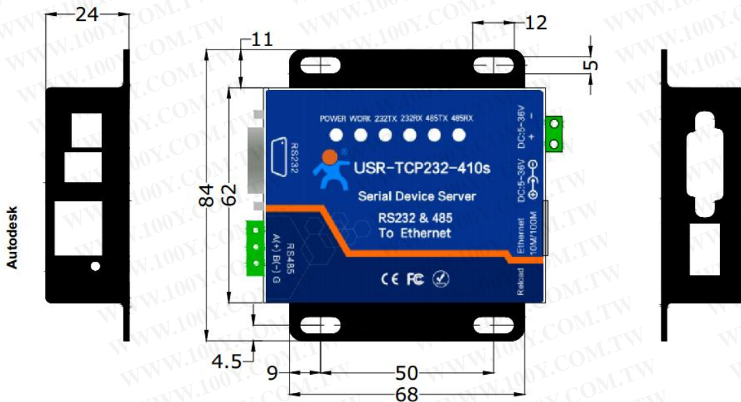
图 4 410S 尺寸图
