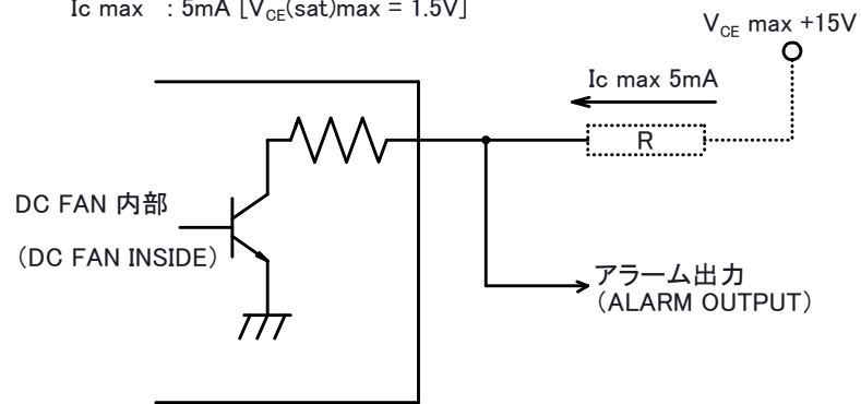
図1 アラーム信号回路 (ALARM SIGNAL CIRCUIT)
