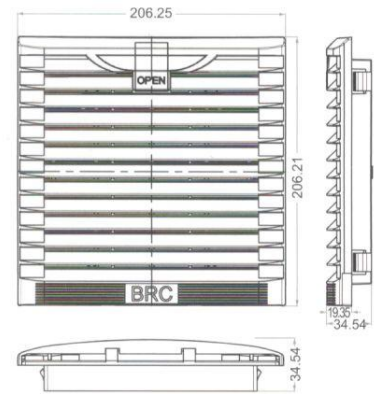
YH-06A For 6 inch fan
