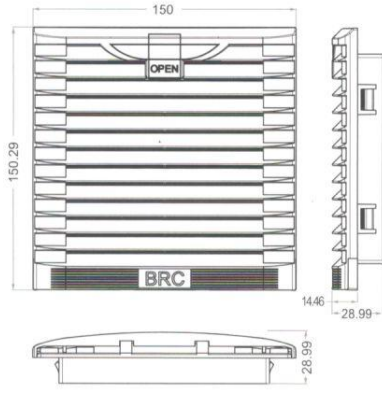
YH-04A For 4 inch fan
