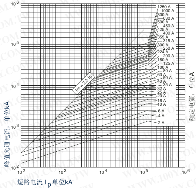
限流曲线
