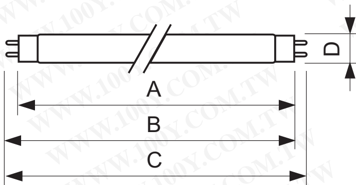
TL-D 18W/54-765 1SL
