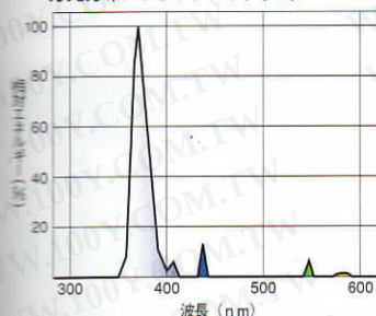
分光分布 ブラックライト (BL)
