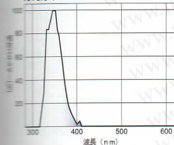
分光分布 ブラックライトブルー (BL-B)
