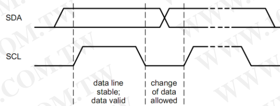
图 6: I 2 C 总线的位传输
