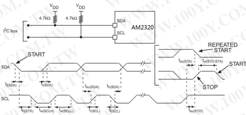
图 13: AM2320 典型的 I2C 总线应用电路和时序图
