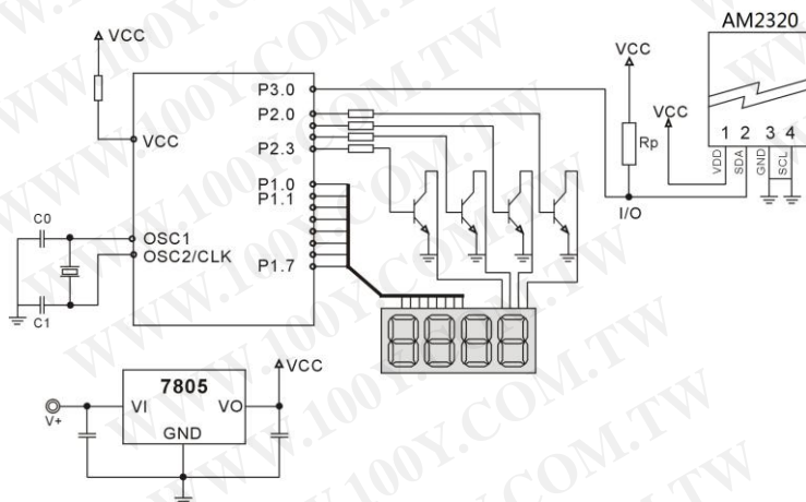
图 19： AM2320 单总线典型电路
