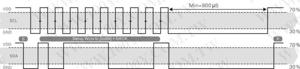
图 15: 唤醒传感器
