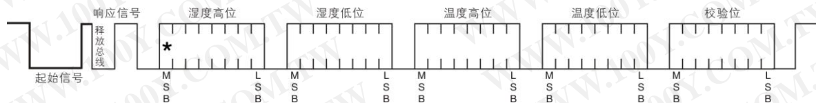
图 20： AM2320 单总线通信协议
