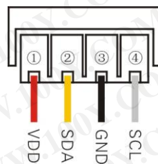
图 4: AM2320 接线图
