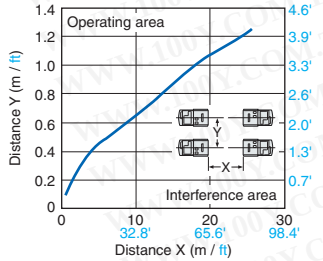
PZ-G51
