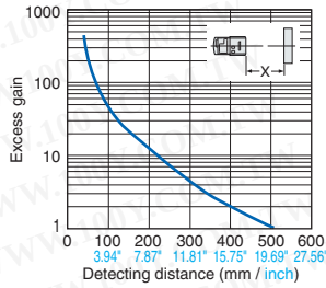
PZ-G101
