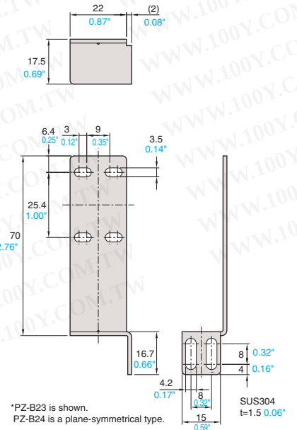
PZ-B23/B24
