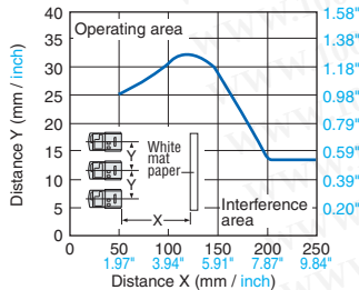
PZ-G101
