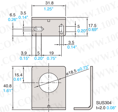
PZ-B03
