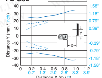
PZ-G62
