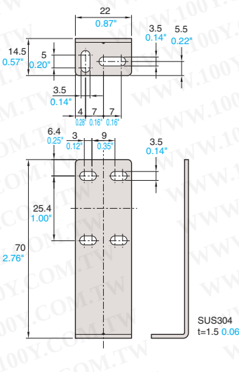
PZ-B02
