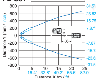
PZ-G51
