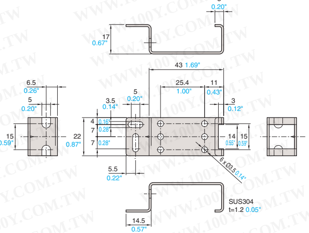
PZ-B11
