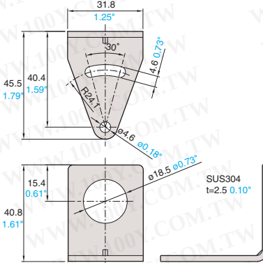
PZ-B04
