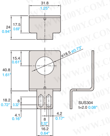
PZ-B25
