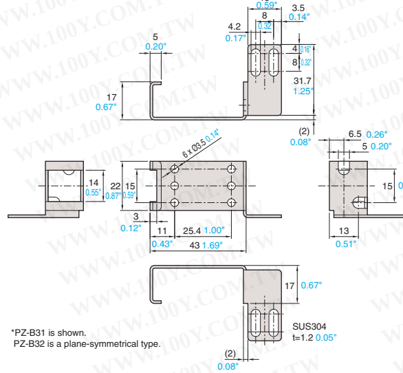
PZ-B31/B32
