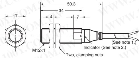
E2A-M12KS04-WP-□□
