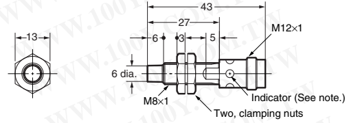
E2A-S08KN04-M1-□□ E2A-M08KN04-M1-□□
