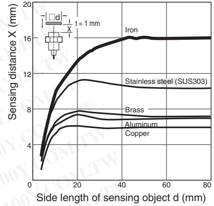
E2A-M18□N16
