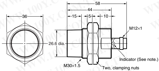
E2A-M30KN20-M1-□□
