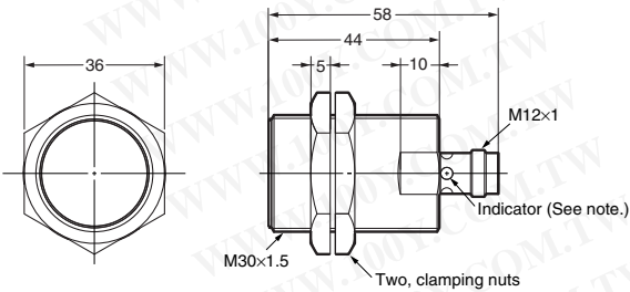
E2A-M30KS15-M1-□□
