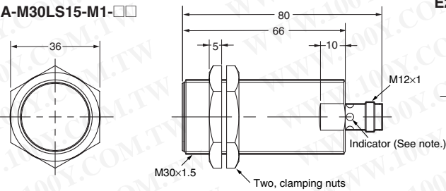
E2A-M30LS15-M1-□□
