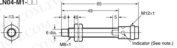
E2A-S08LN04-M1-□□ E2A-M08LN04-M1-□□
