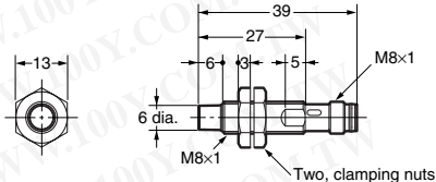
E2A-S08KN04-M5-□□
