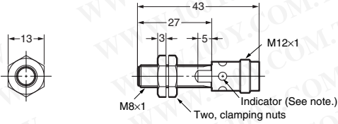
E2A-S08KS02-M1-□□ E2A-M08KS02-M1-□□
