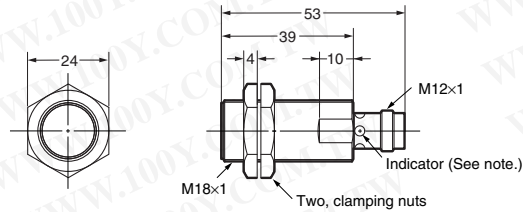
E2A-M18KS08-M1-□□
