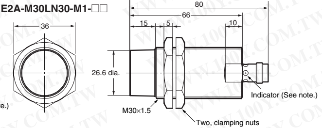
E2A-M30LN30-M1-□□
