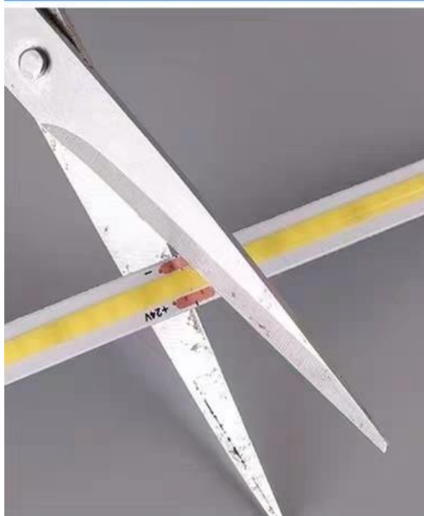
1.如图在铜焊盘中间 有一条黑线 沿线剪开
