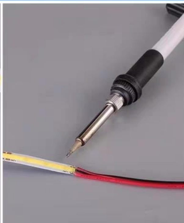
2.裁剪完后，在铜焊盘位置上锡 然后将线头置于锡堆上
