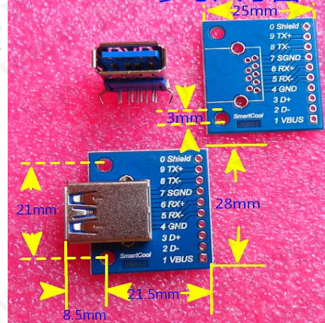
USB3.0-AF参考尺寸图：
