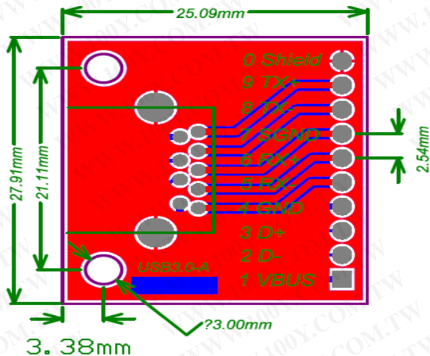
USB3.0-AF参考尺寸图：
