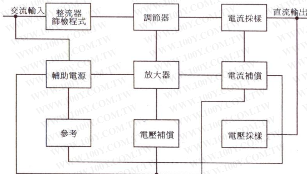
Fig.1 電路圖
