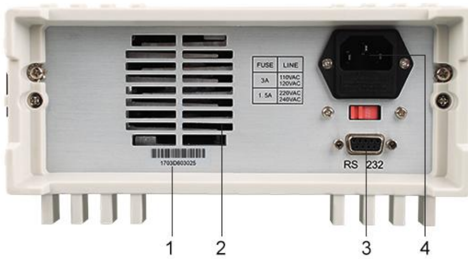
图3.2 TD1000系列电源的后面板
