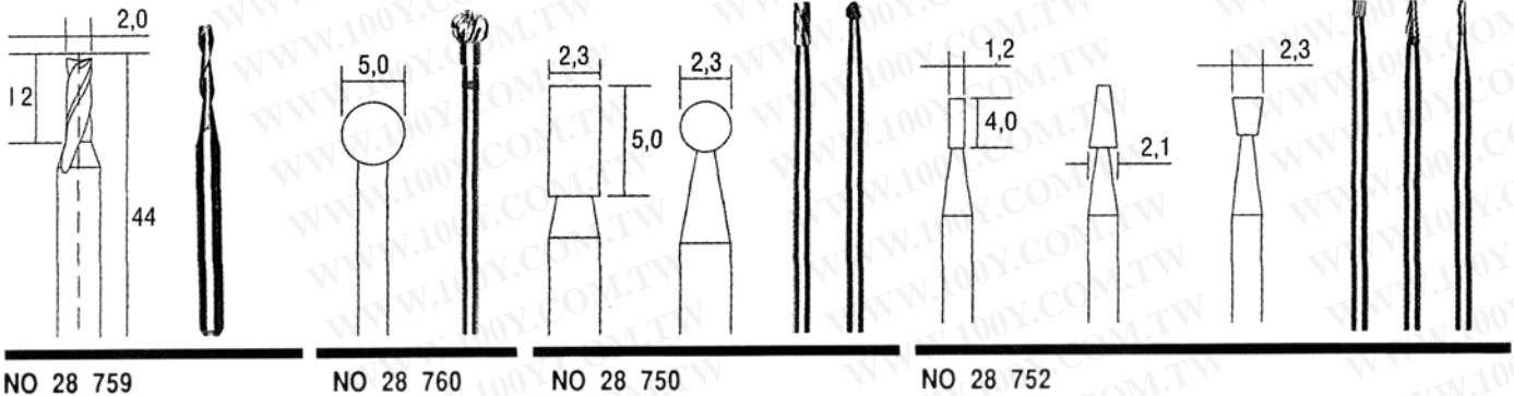
NO 28 759 超硬鋼銑刀
