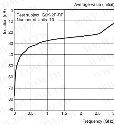
G6K-2F-RF
